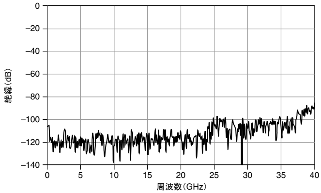
図 2. 標準絶縁
