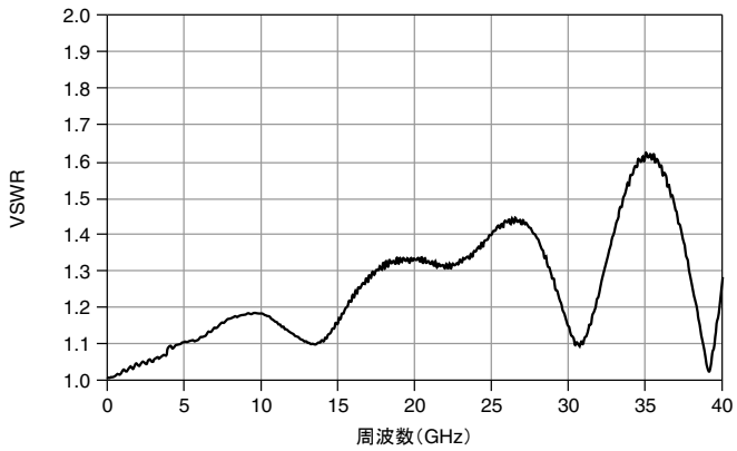
図 3. 標準 VSWR
