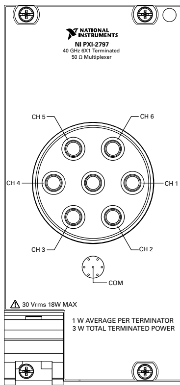
図 5. NI 2797 フロントパネル
