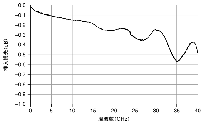
図 1. 標準挿入損失
